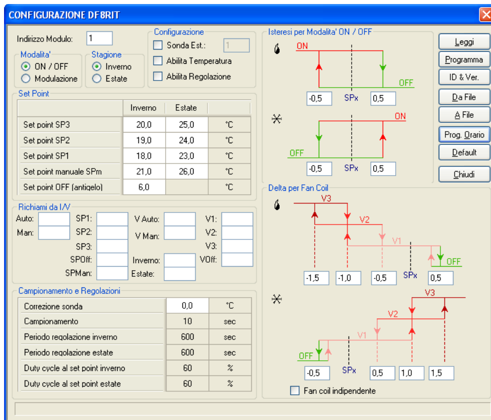
Figura 1: Configurazione controllo di temperatura
