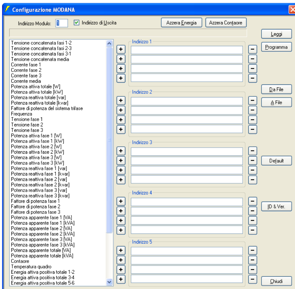
Figura 1: Pannello di configurazione modulo ModANA
