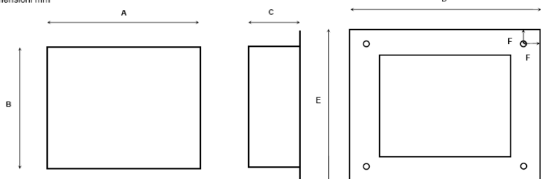
Scatola da incasso per Touch Screen Dimensioni mm
